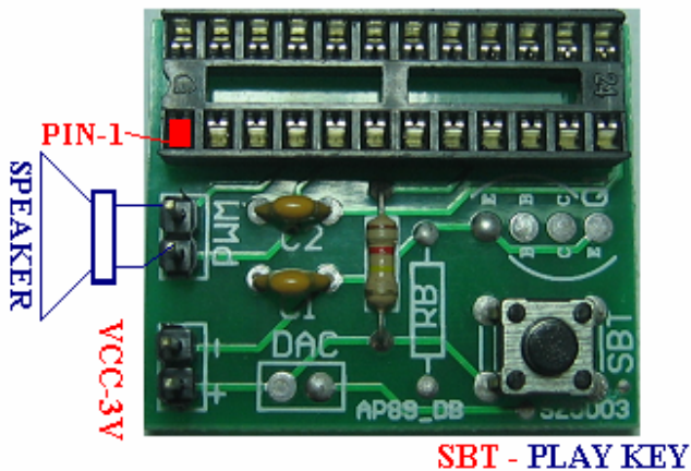
Part No. : AP89XS-DBP
