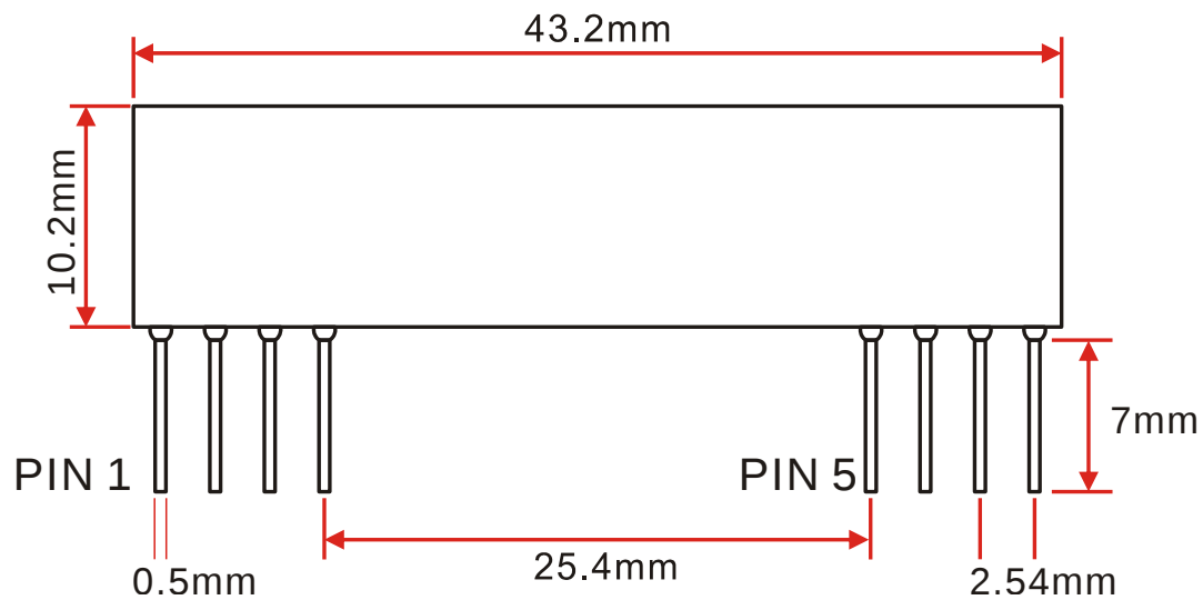
尺寸圖
