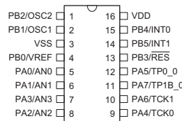
HT66F15 16 DIP-A/NSOP-A/SSOP-A
